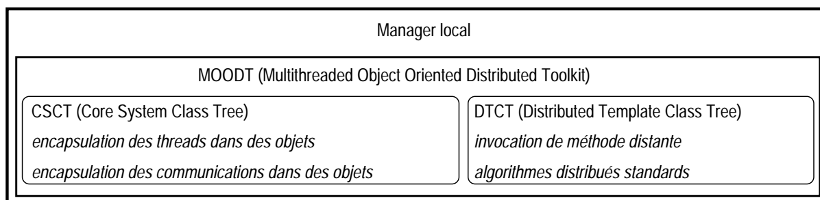
Fig. 8.2 Structure interne du Manager local
