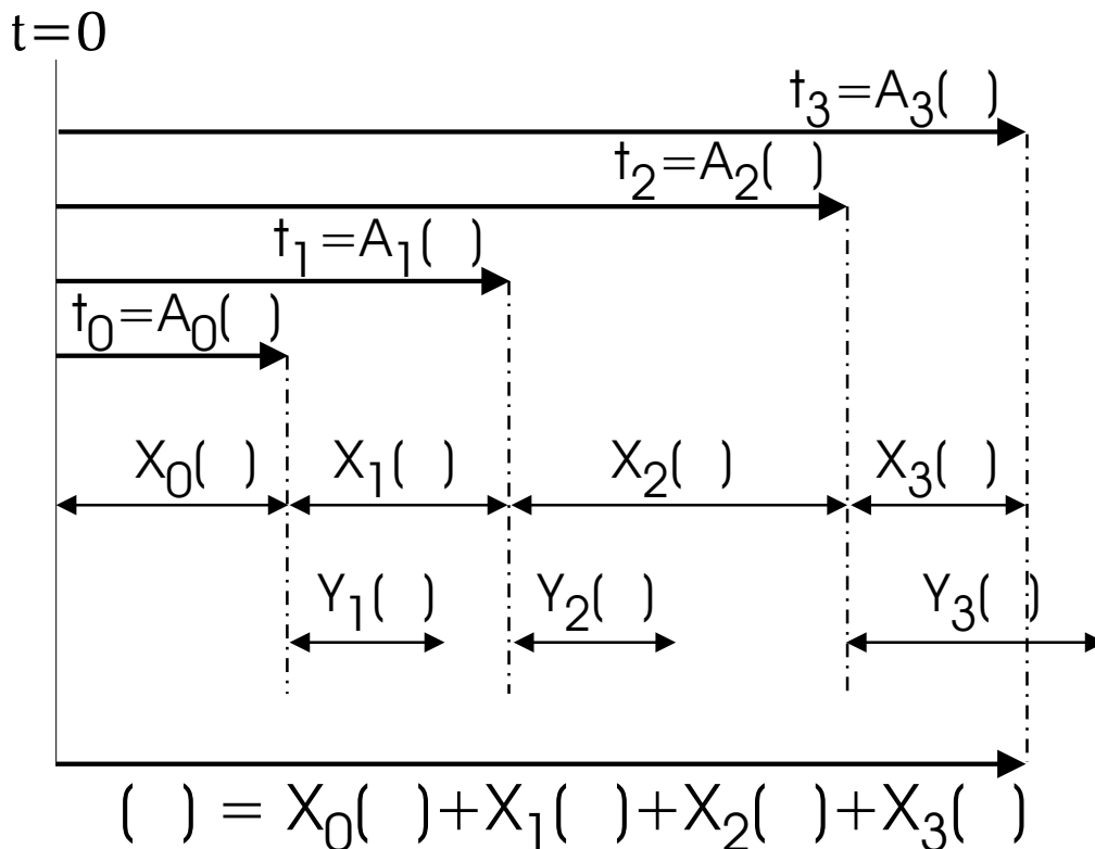
Fig. 10.1 Exemple de double-faute
