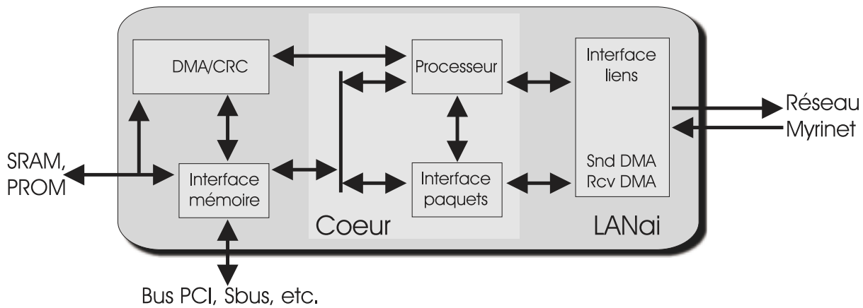
Fig. 3.2 LANai
