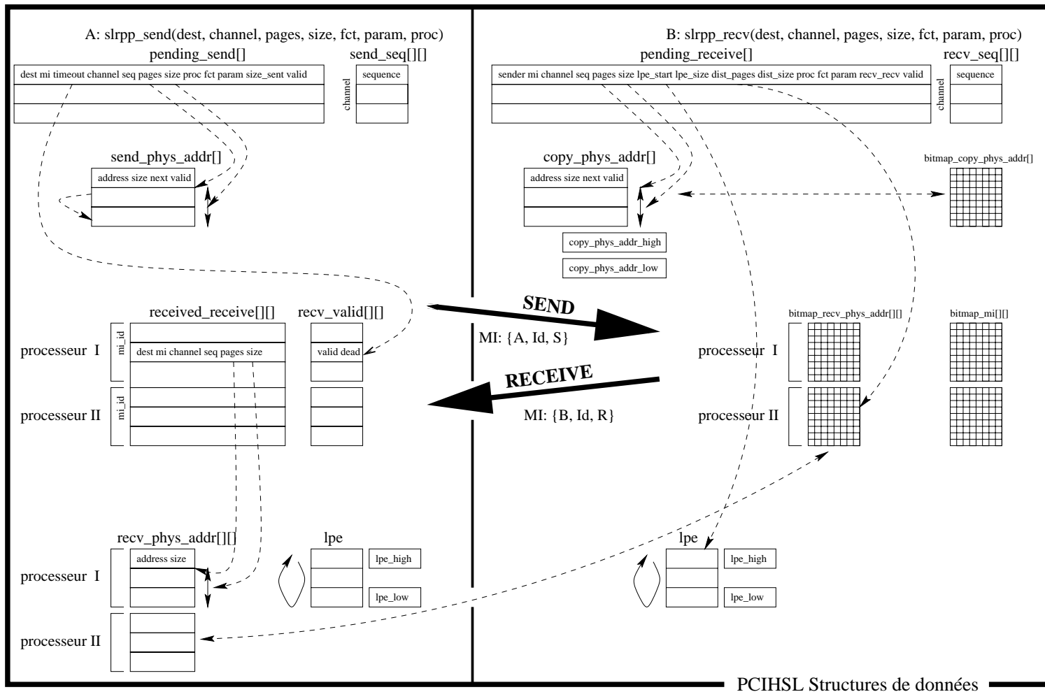
Fig. D.1 Structures de données en jeu dans SLRP/P
