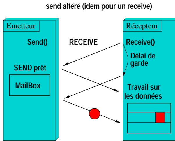
Fig. 6.4 Travail sur des données altérées
