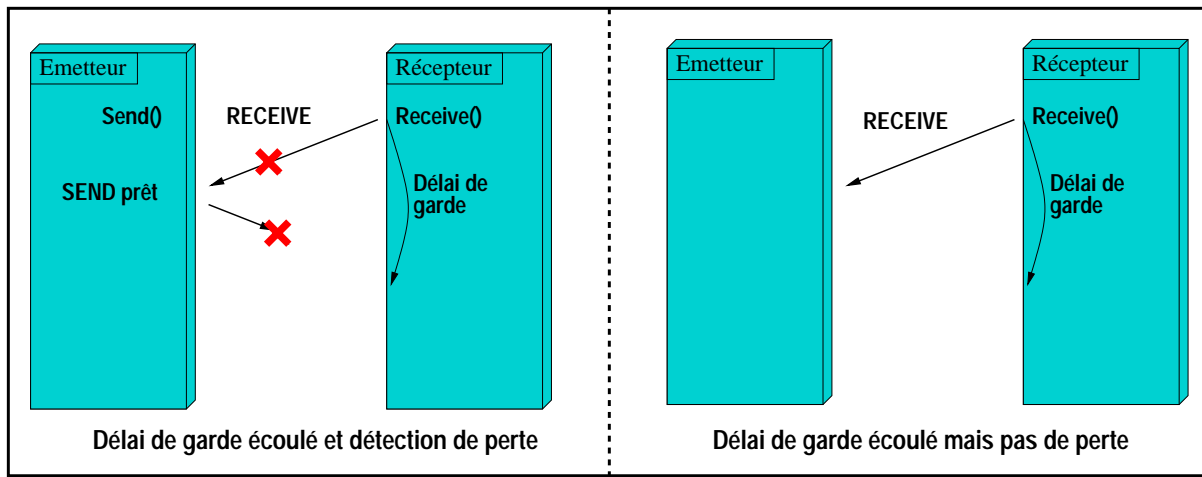
Fig. 6.3 Délai de garde
