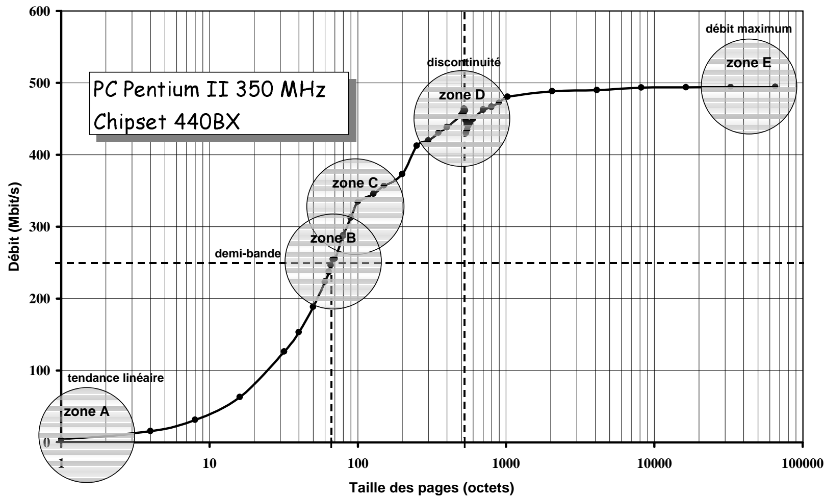
Fig. 9.2 Cinq zones singulières
