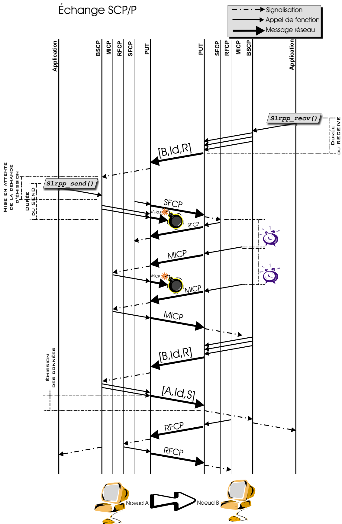
Fig. 6.10 Échange SCP/P avec fautes (et slrpp_send() après slrpp_recv() )
