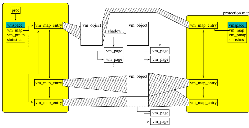
Fig. 7.2 Référencement dans la carte de protection
