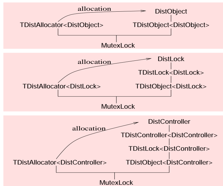
Fig. 8.10 Objets distribués et allocateurs
