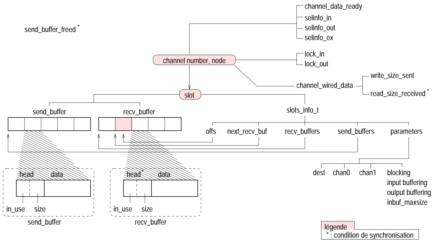
Fig. E.1 Structures de données en jeu dans MDCP
