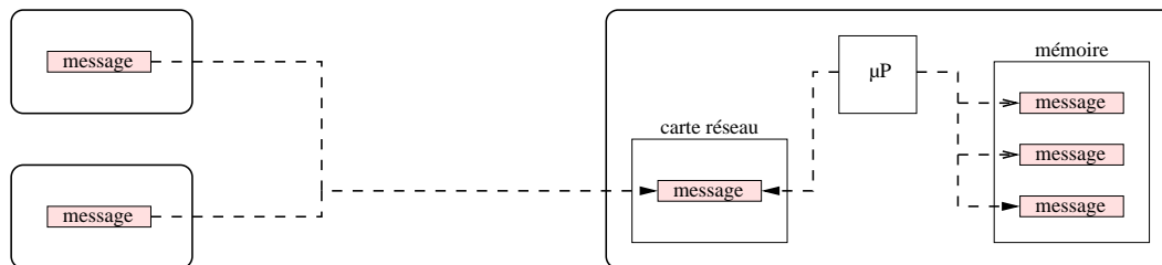
Fig. 2.3 Dépôt de données à travers une carte réseau traditionnelle
