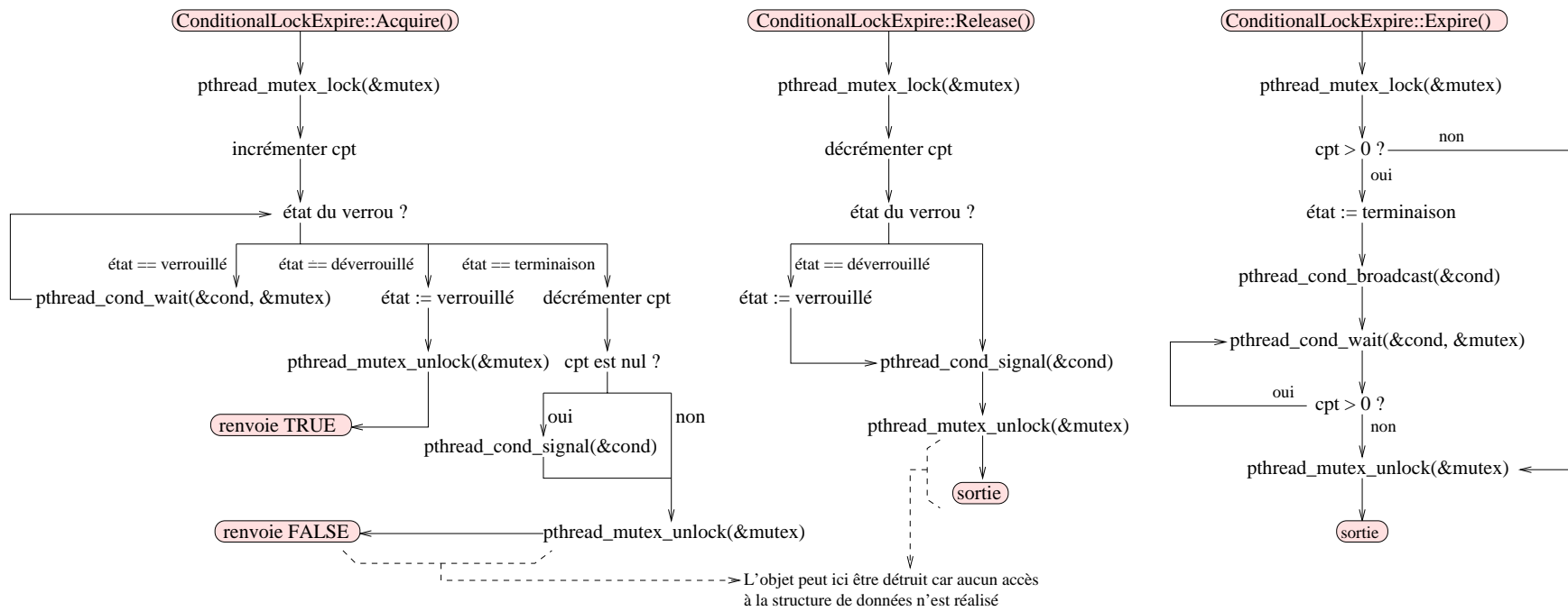
Fig. 8.5 Organigramme de l'algorithme de verrouillage
