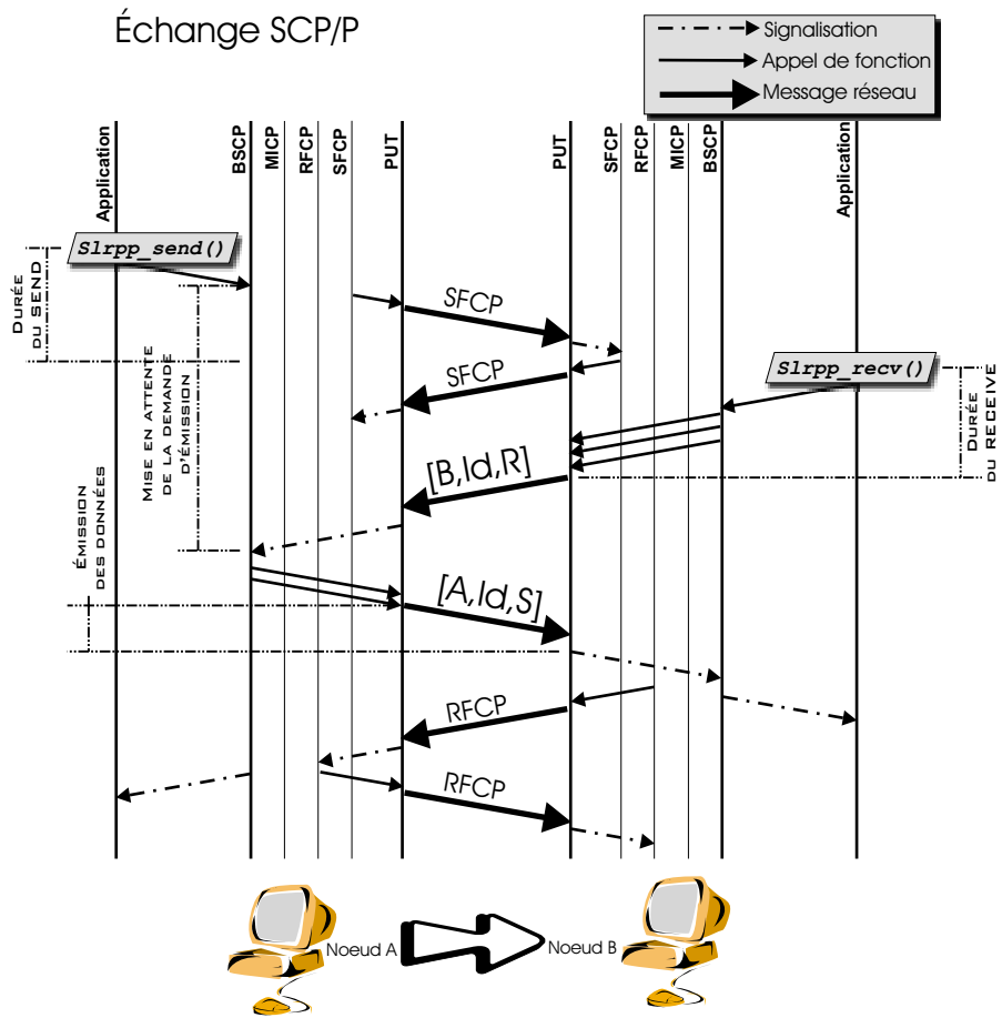
Fig. 6.9 Échange SCP/P sans faute (et slrpp_send() avant slrpp_recv() )
