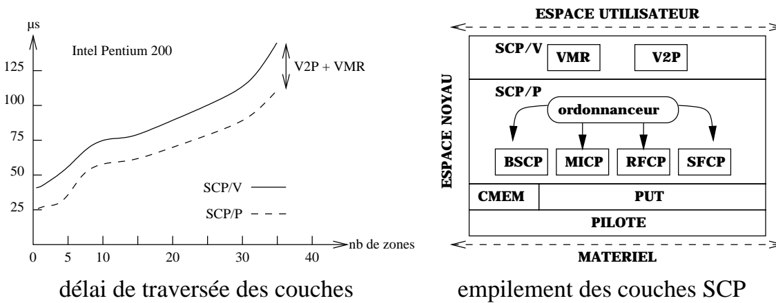
Fig. 9.8 Performances des couches sécurisées haut-niveau
