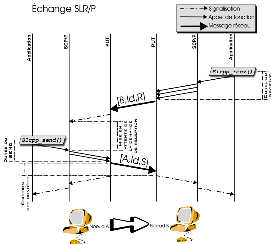
Fig. 5.3 Échange SLR/P : slrpp_send() après slrpp_rcv()
