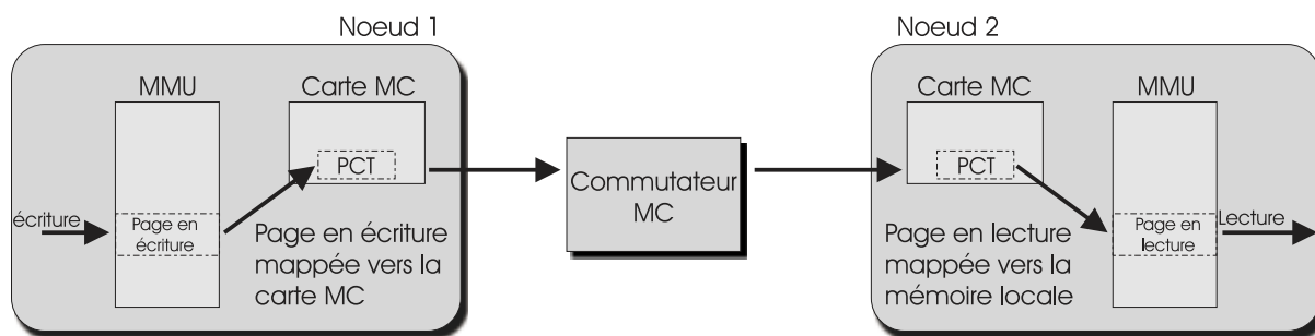
Fig. 3.1 Transfert de données avec Memory Channel
