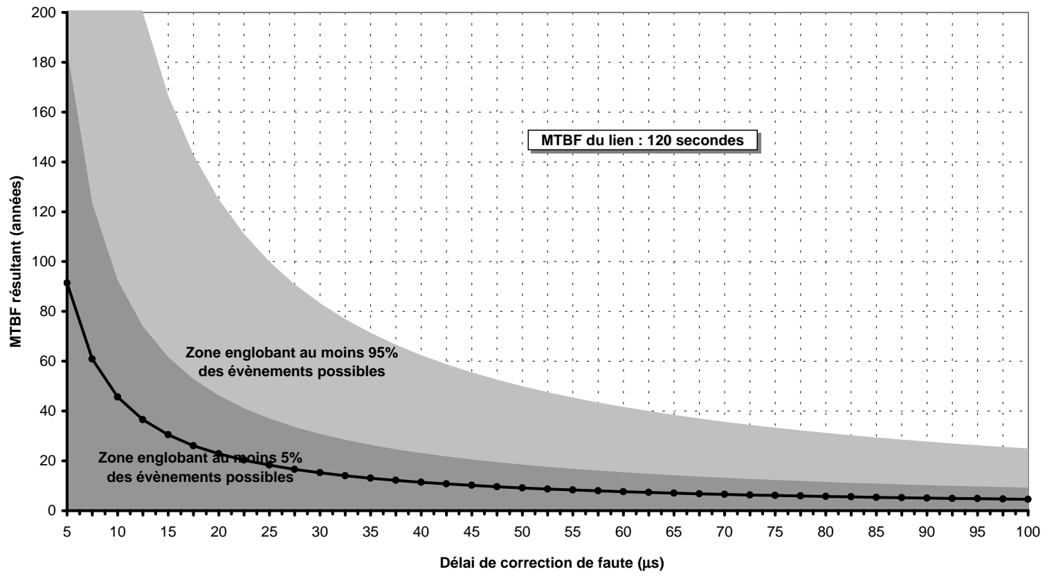
Fig. 10.4 Dispersion des événements de double-faute
