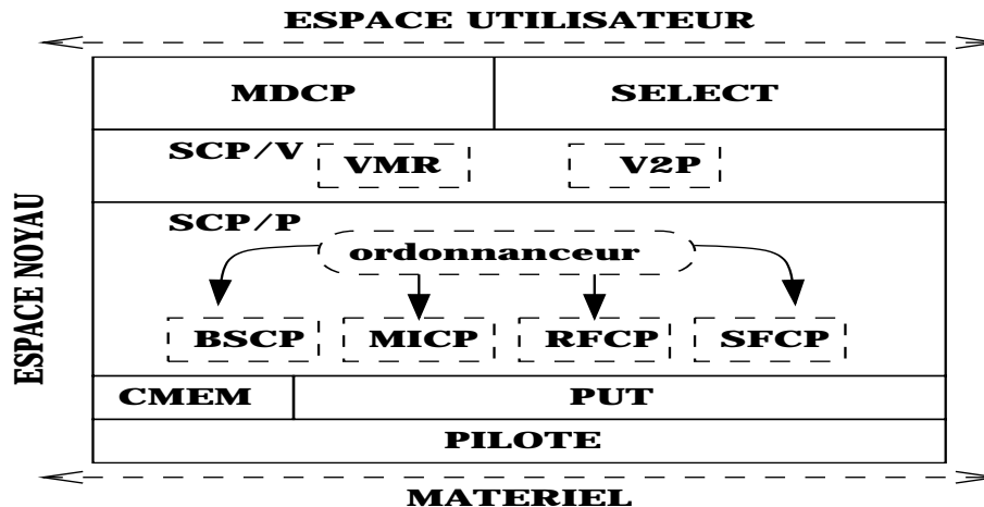
Fig. 7.5 Protocoles noyau
