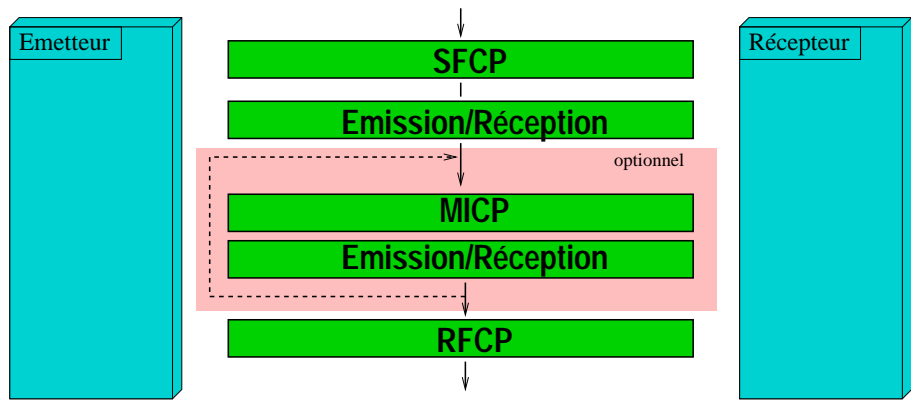
Fig. 6.8 Enchaînement des opérations
