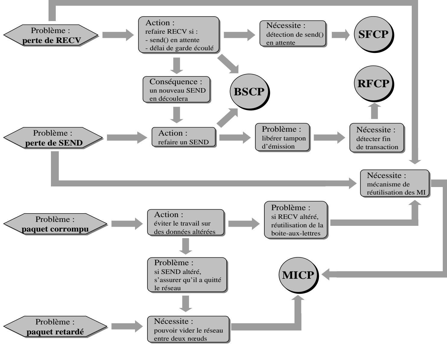
Fig. 6.5 Conception du protocole
